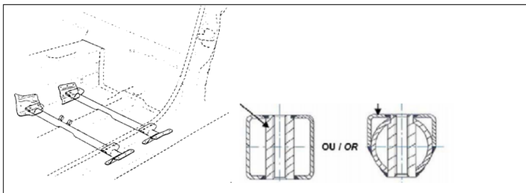
Рис. 1. Крепление сидений.
