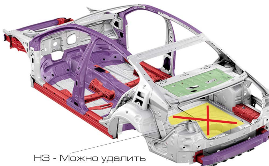
Рис. 4. Общая схема силовой структуры кузова.
