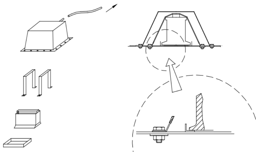
Рис.3. Крепление аккумуляторной батареи.
