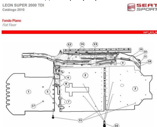
Рис. 8.3. Плоское дно.
