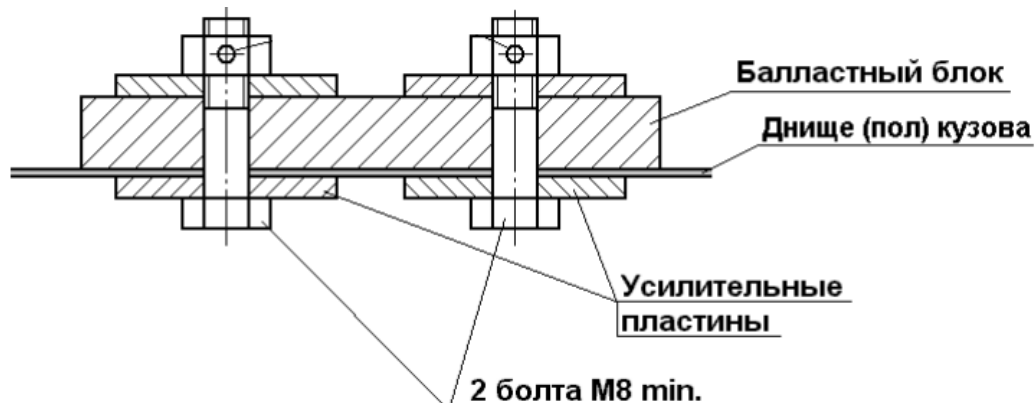
Рис. 5.2. Крепление балласта.
